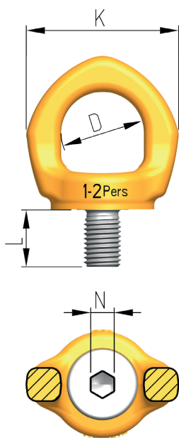
Abb. 2: Maßzeichnung PSA INOX-STAR für 1-2 Personen
