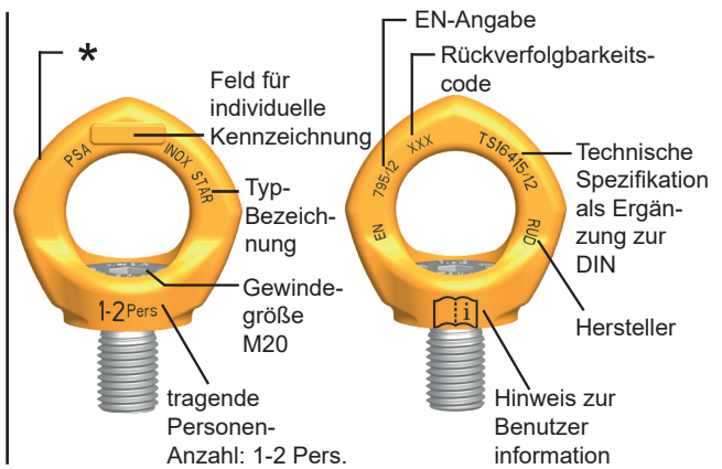
PSA INOX-STAR für 1-2 Personen (M20)
