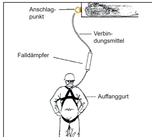
Abb. 1: Übersicht Auffangsystem mit Falldämpfer (Quelle: BGR/GUV-R 198, 03/2011, S. 13 Bild 7)
