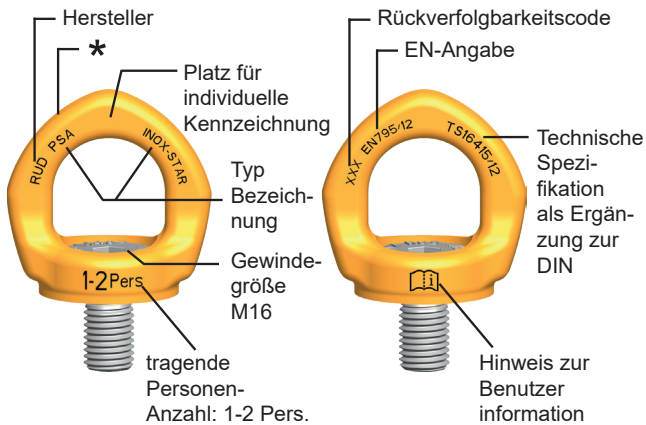
PSA INOX-STAR für 1-2 Personen (M16)
