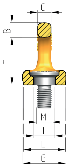
Abb. 2: Maßzeichnung PSA INOX-STAR für 1-2 Personen
