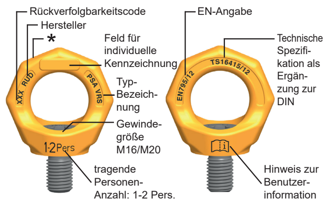
PSA VRS für 1-2 Personen (M16 / M20)
