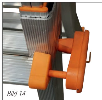
Bild 14 Sperrelement entriegelt
