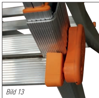
Bild 13 Sperrelement gesichert
