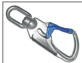
IKV 21 (EN 362:2004-T) mit Fallanzeiger
