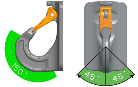
Bild 1. zulässige Belastungsrichtungen
